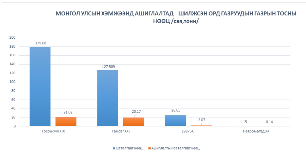
Зураг-6: Газрын тосны нөөц
