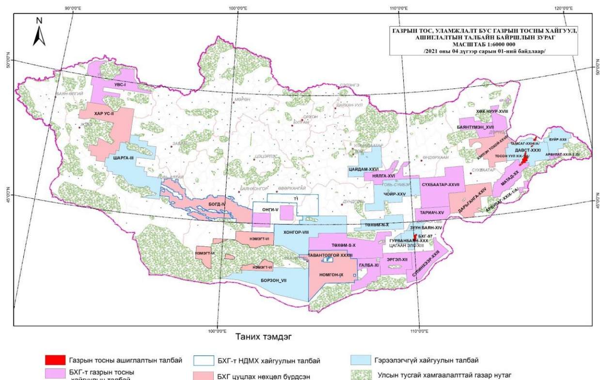
Зураг-1: Газрын тосны хайгуул, ашиглалтын талбайн зураглал
